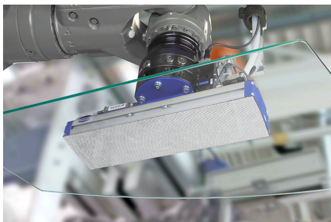
Sistema de ventosas FXP con capa protectora SU para la manipulación de cristal
