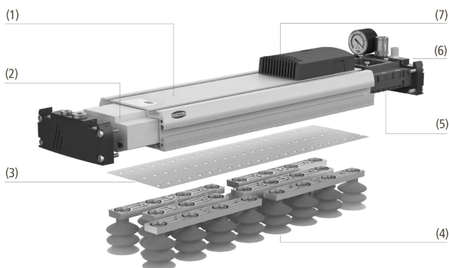
Diseño del sistema Sistemas de planos aspirantes FXP
